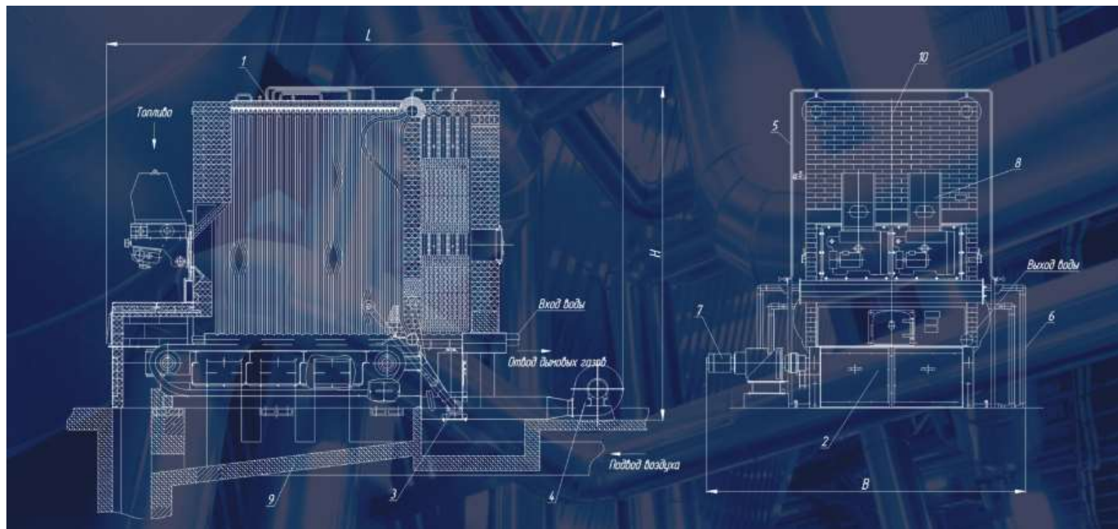
Рис. 1. Котел водогрейный серии КВ-ТС. 1. Блок котла; 2. Топка котла (ТЛЗМ или ТЧЗМ); 3. Система возврата уноса; 4. Вентилятор острого дутья; 5. Трубопроводы воздушные; 6. Трубопроводы дренажные; 7. Привод топки; 8. Забрасыватели топки; 9. Фундамент котла; 10. Изоляция и обшивка котла.
